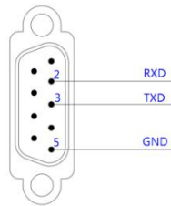
COM1,2-RS232 接口定义
