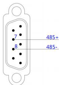
COM3-RS485
