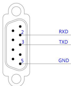
COM1,2,3,4-RS232 接口定义
